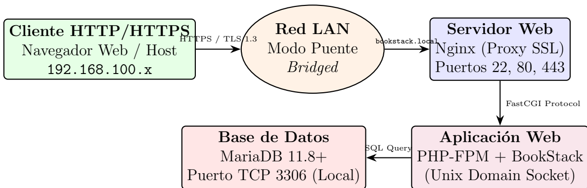
Figura 1: Diagrama de arquitectura .As Built" de 3 capas con terminación TLS y Hardening de Firewall.
